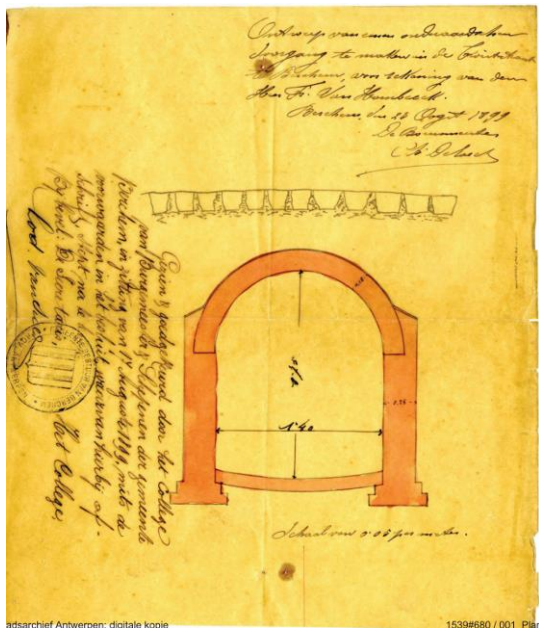
Foto 24 Ontwerptekening onderaardse gang van 1899
